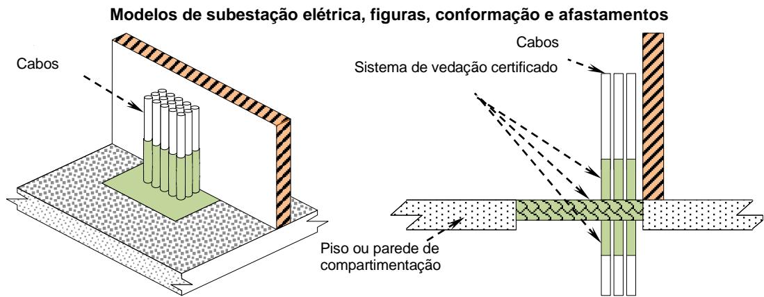
Figura A.1: Exemplo de vedação de abertura para passagem de cabos entre ambientes compartimentados
